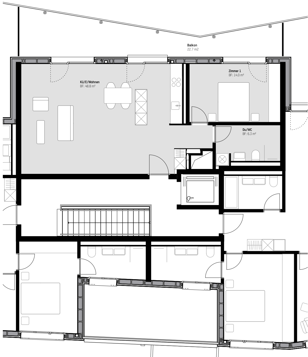
2.5 Zimmerwohnung Wohnfläche 69.2 m 2 (Innenkante Umfassungswände)
